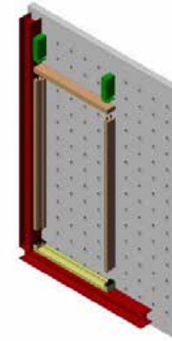
Ingepakte dorpel in de opsluitbank
