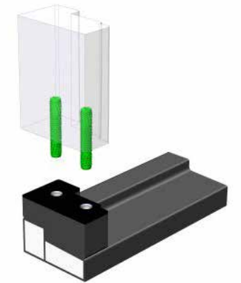
NEO-FIX: NEO-dorpel inclusief FastFix deugel
